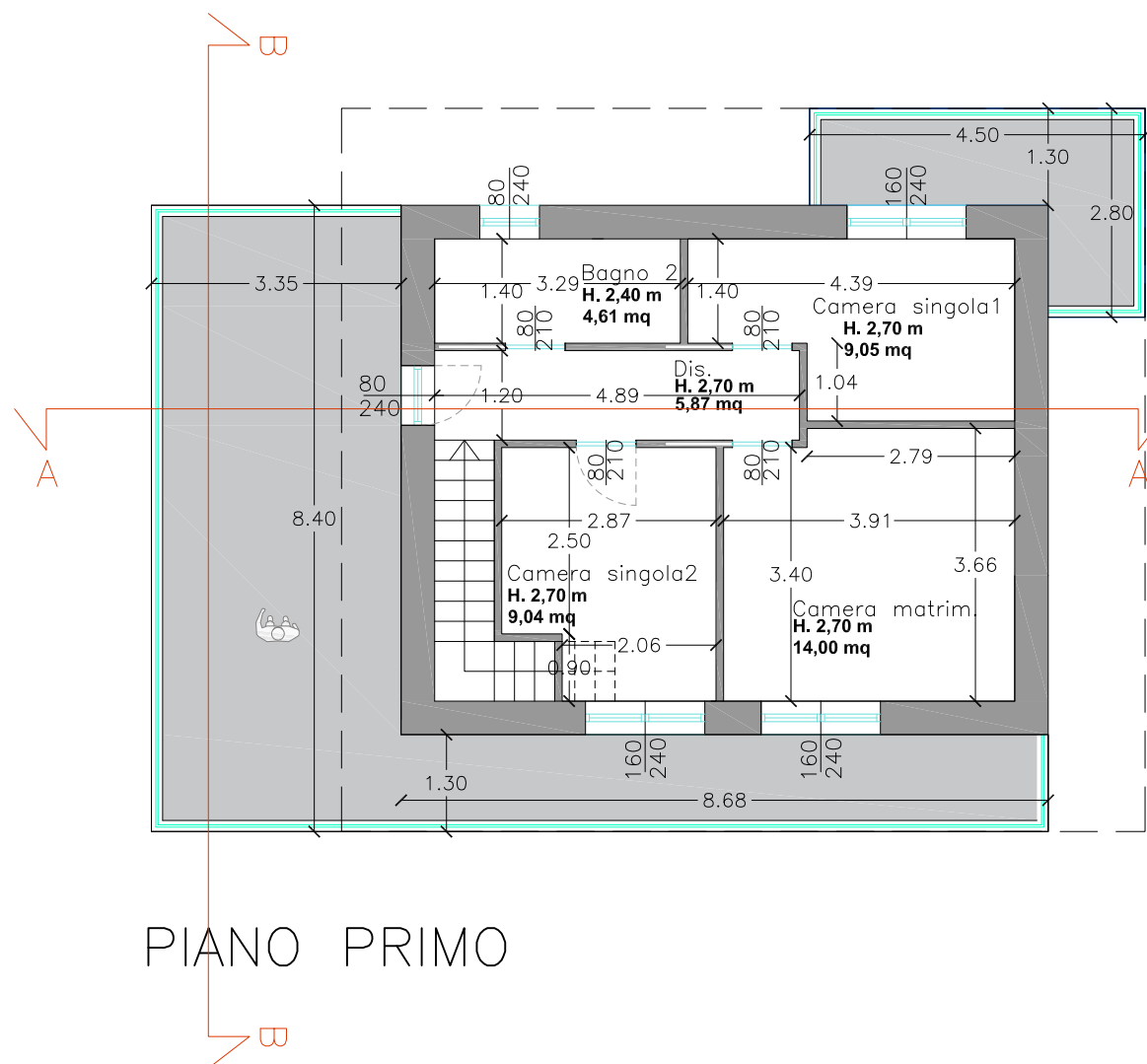
PIANO PRIMO
